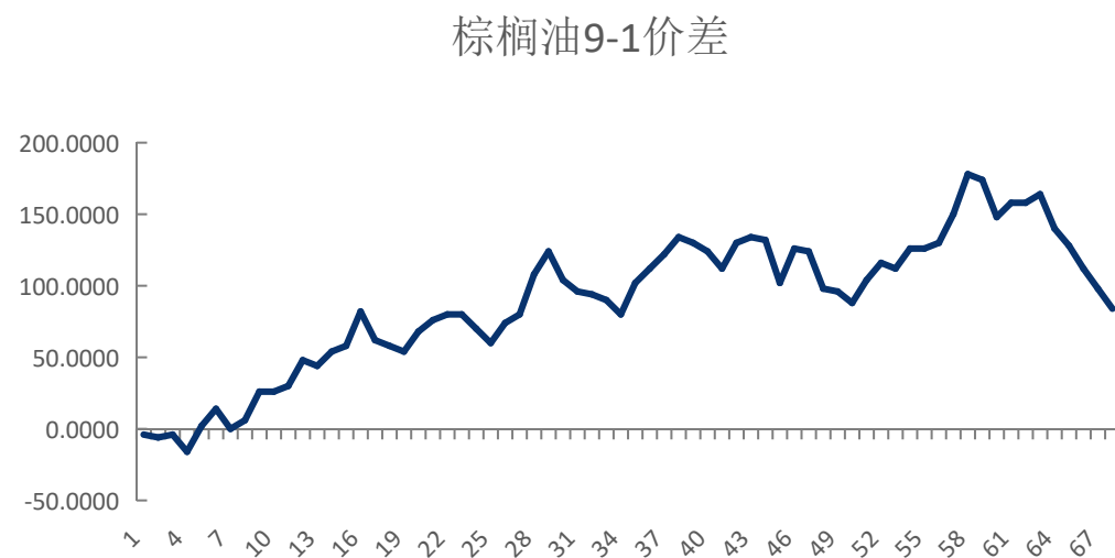
图3、棕榈油9-1价差走势图
