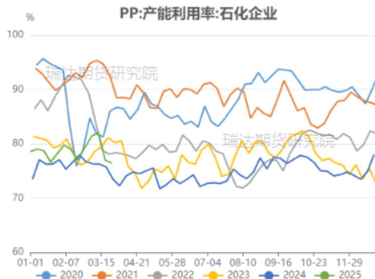
图17、PP生产企业产能利用率
