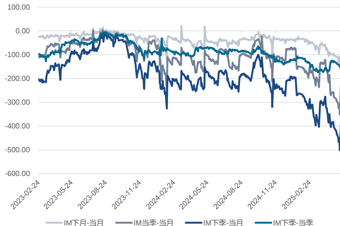
「IM跨期」
