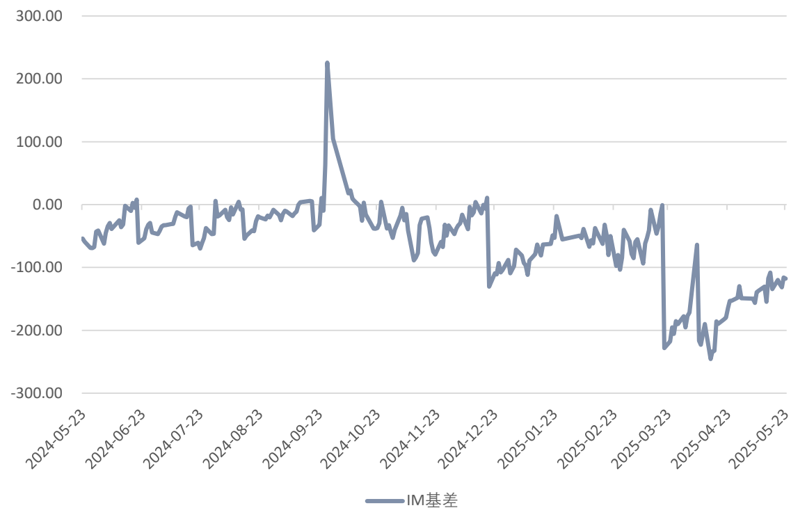
「IM基差」
