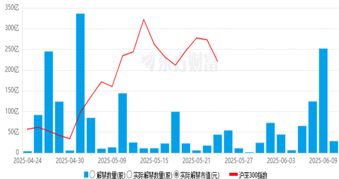
「限售解禁」
