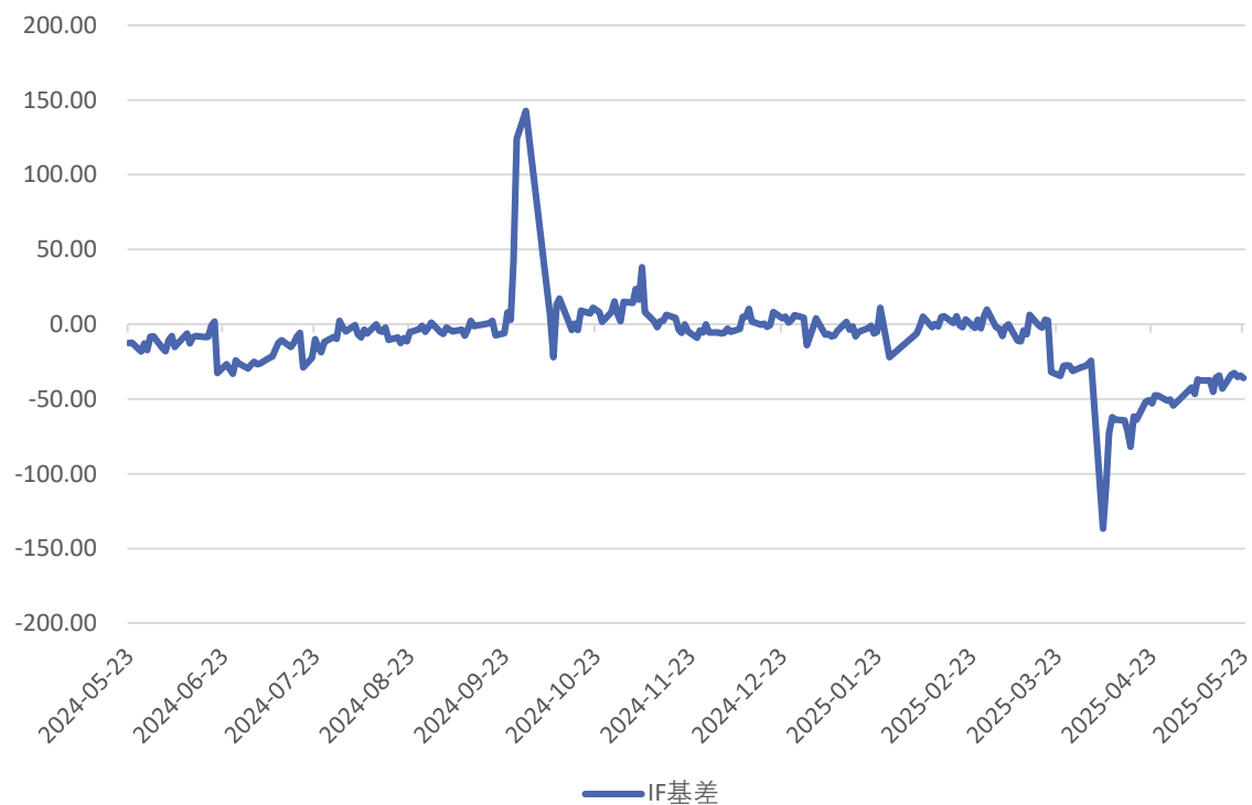
「IF基差」
