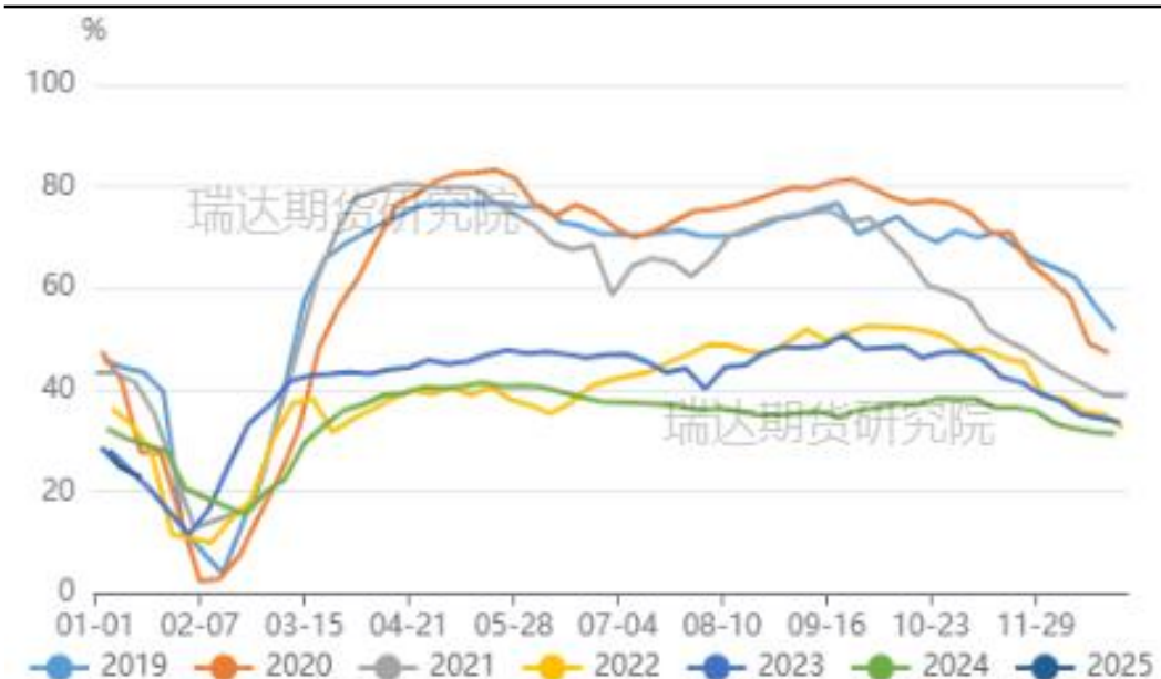
图14、水泥发运率
